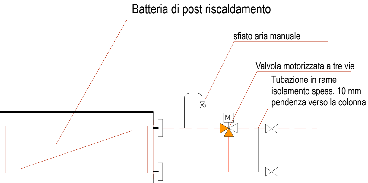
Particolare collegamento batterie di post riscaldamento ad acqua da canale
